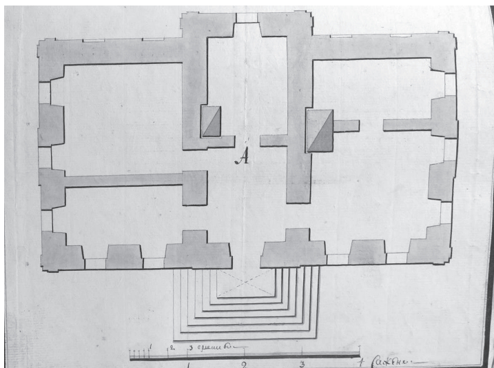
План и фасад каменных покоевъ для хранения денег подушного сбора. Архитектор Пётр Никитин
