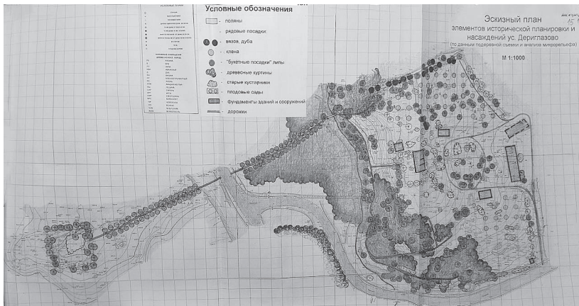
Эскизный план элементов исторической планировки и насаждений усадьбы Дериглазово (по данным подеревной съемки и анализа микрорельефа. Масштаб 1 : 1000) «Центрлеспроект» (Москва, 1998). Архив Пушкинского Заповедника. Научный архив (АПЗ. Н/а)
